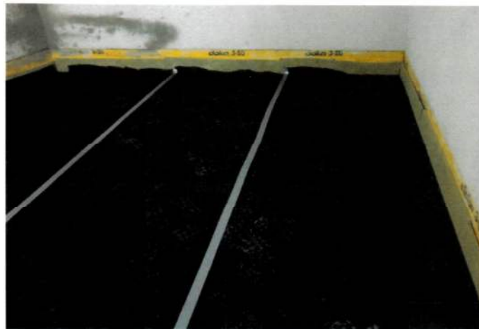
Abbildung A 2.1: Montagesituation mit Trittschalldämmmatten und Randdämmstreifen, Stöße mit Klebeband
